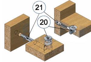
Эксцентриковая стяжка
