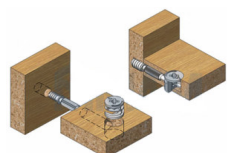
Эксцентриковая стяжка
