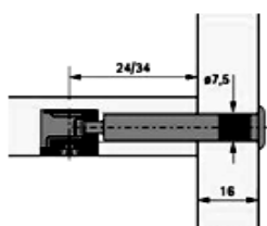
Дюбель концевой
